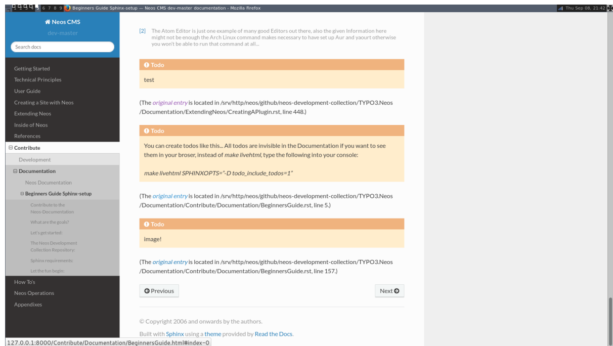
Fig. 4: Sphinx todoclist
